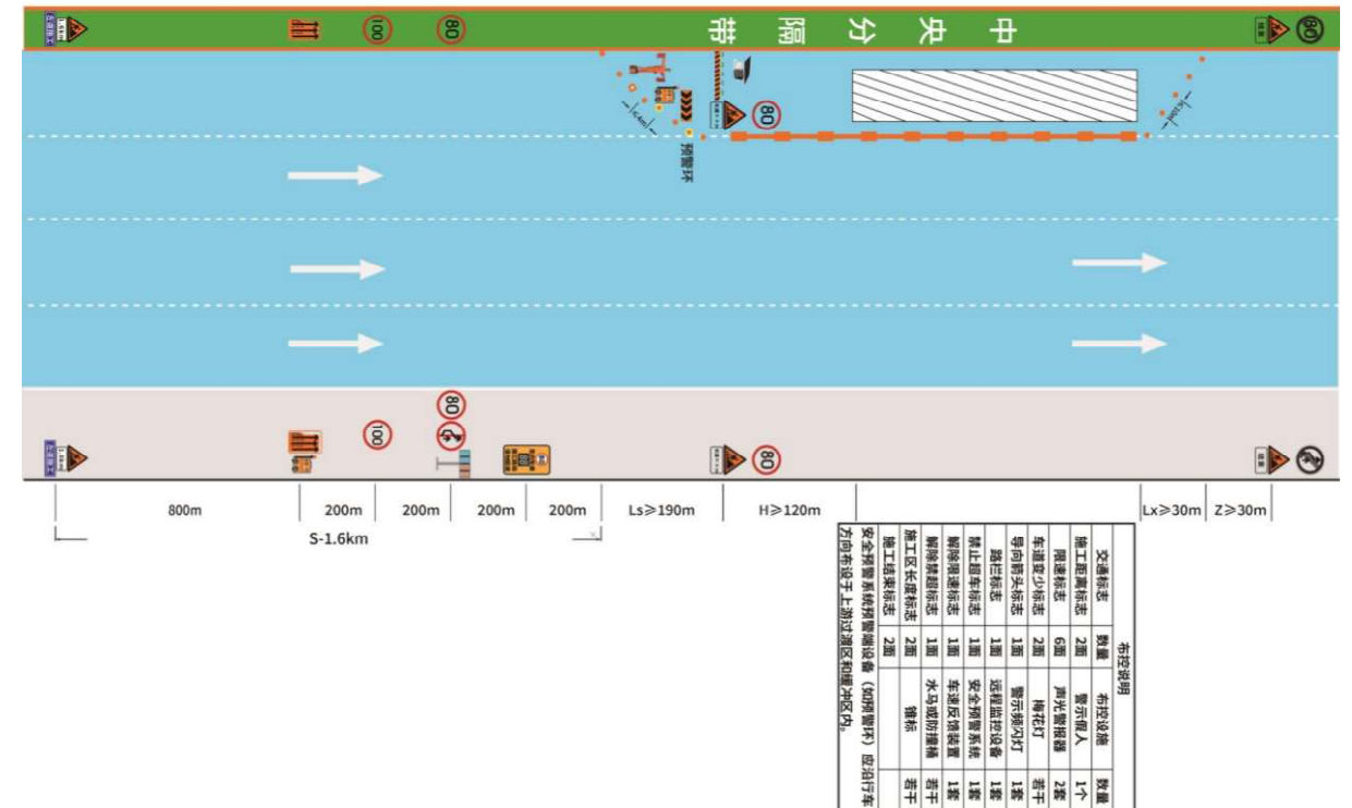
图 8-5 八车道封闭内侧 1 车道养护作业
