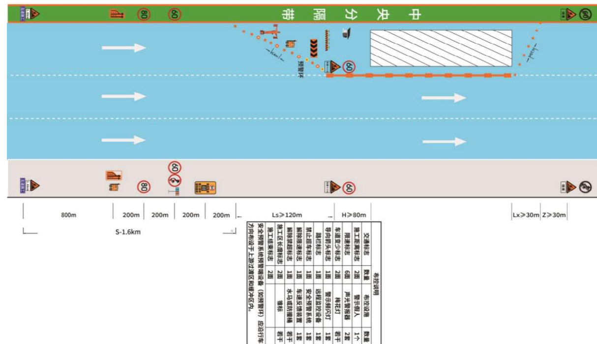
图 8-3 六车道封闭内侧 1 车道养护作业
