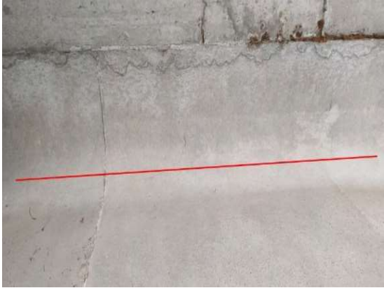
图 3-2：东园互通 D 匝道桥 6—4T 梁：距 5 号墩 0m 处，左侧，翼板与腹板交接处纵向裂缝；数量：1 条，长度：1.5m，宽度：0.14mm。
