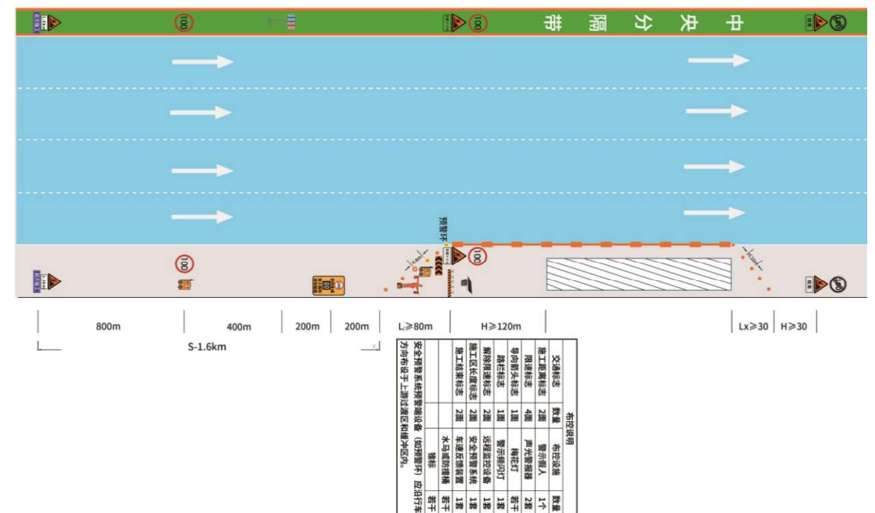
图 8-6 八车道封闭路肩养护作业
