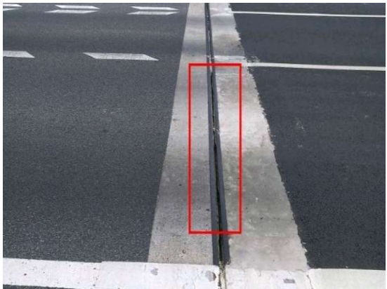
图 3-22 海澄主线分岔主线左线 1 号桥(上行) 6f 伸缩缝: 距右侧 3m 处, 伸缩缝橡胶条橡胶带老化破损; 数量: 1 处, 长度: 3m, 宽度: 0.02m。
