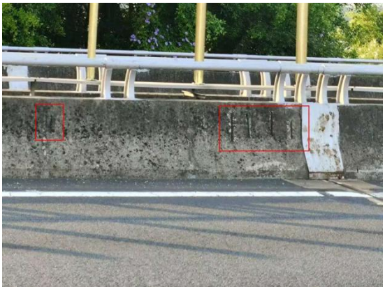
图 3-21 尖石山中桥(上行) HL-L-1 栏杆、护栏: 胀裂剥落; 数量: 5 处, 长度: 0.2m 宽度: 0.1m。
