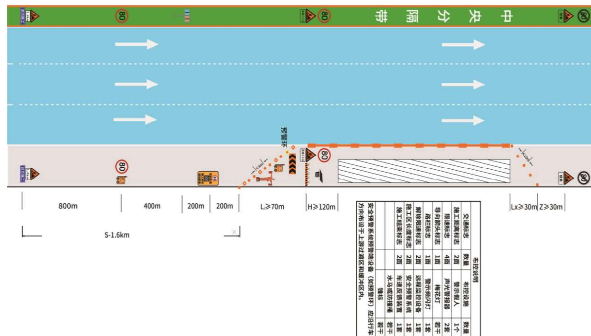
图 8-4 六车道封闭路肩养护作业
